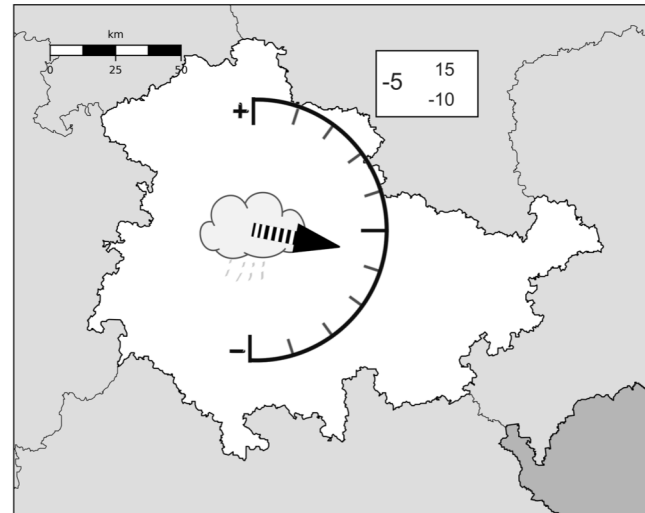
Sommerniederschlag
