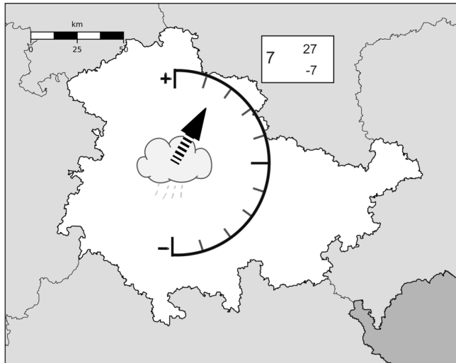
Jahresniederschlag
