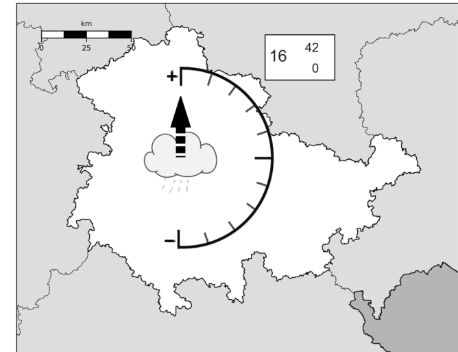
Winterniederschlag
