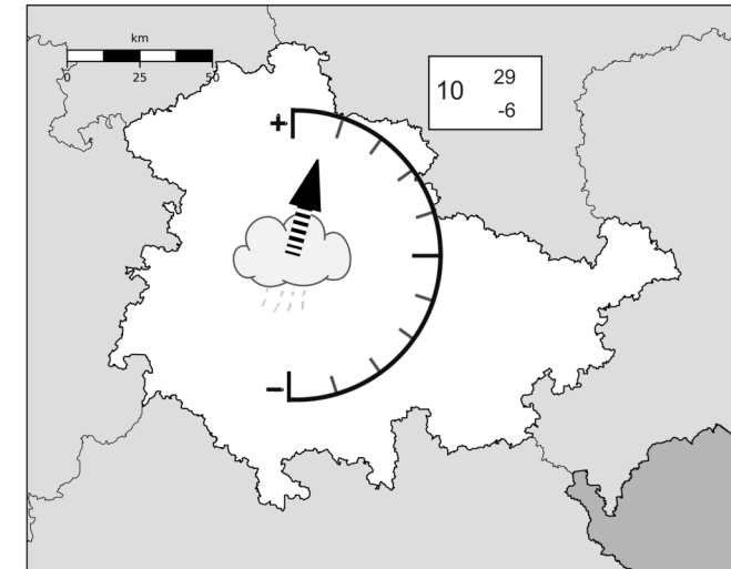
Winterniederschlag
