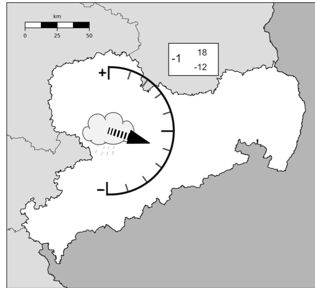
Sommerniederschlag
