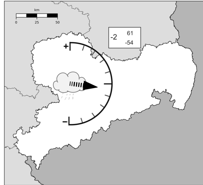
Sommerniederschlag
