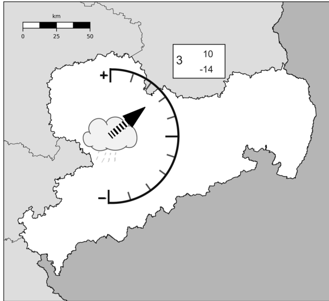
Jahresniederschlag
