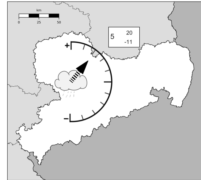
Winterniederschlag
