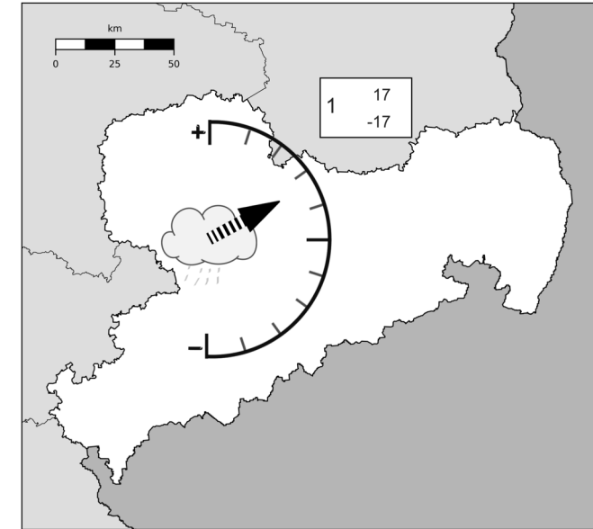
Winterniederschlag
