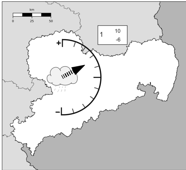
Jahresniederschlag
