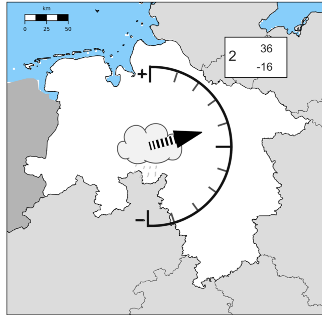
Sommerniederschlag
