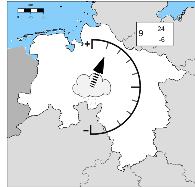
Winterniederschlag
