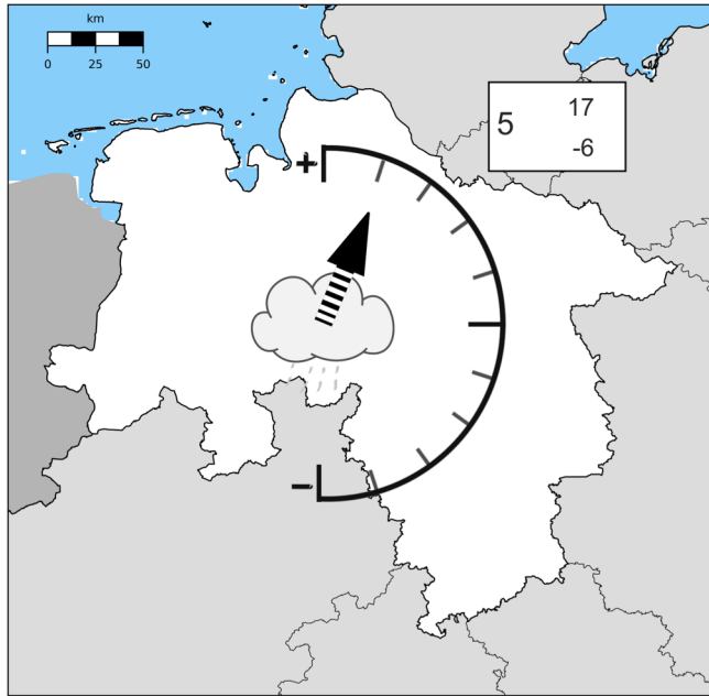
Jahresniederschlag
