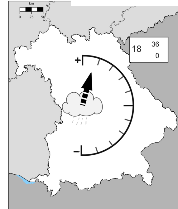
Winterniederschlag
