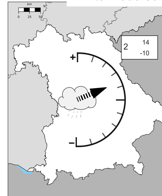
Winterniederschlag
