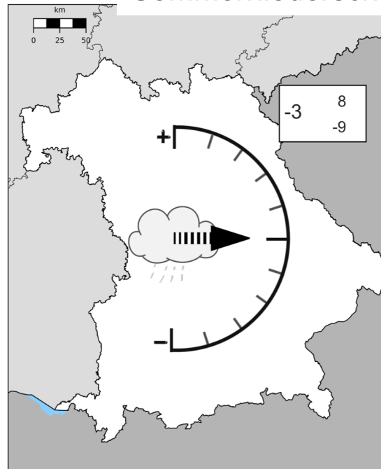
Sommerniederschlag
