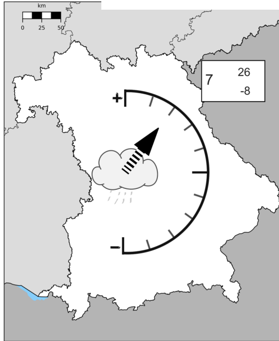
Jahresniederschlag
