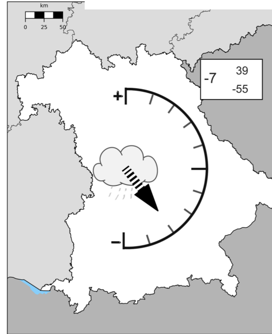
Sommerniederschlag
